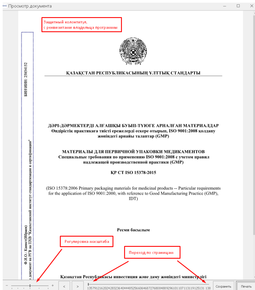
Рисунок 6 – Просмотр документов
