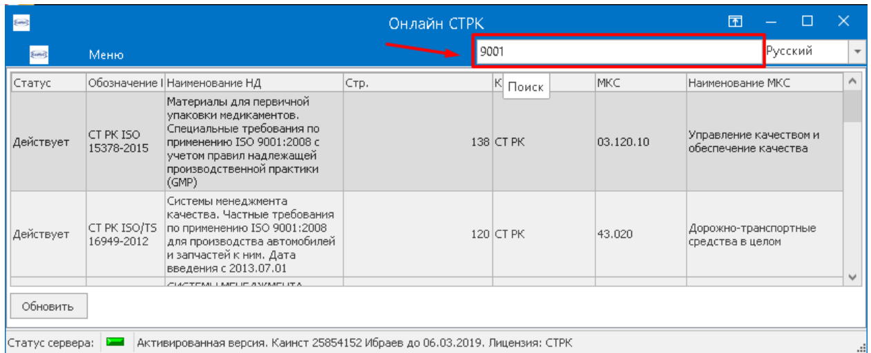
Рисунок 5 – Поиск документов
