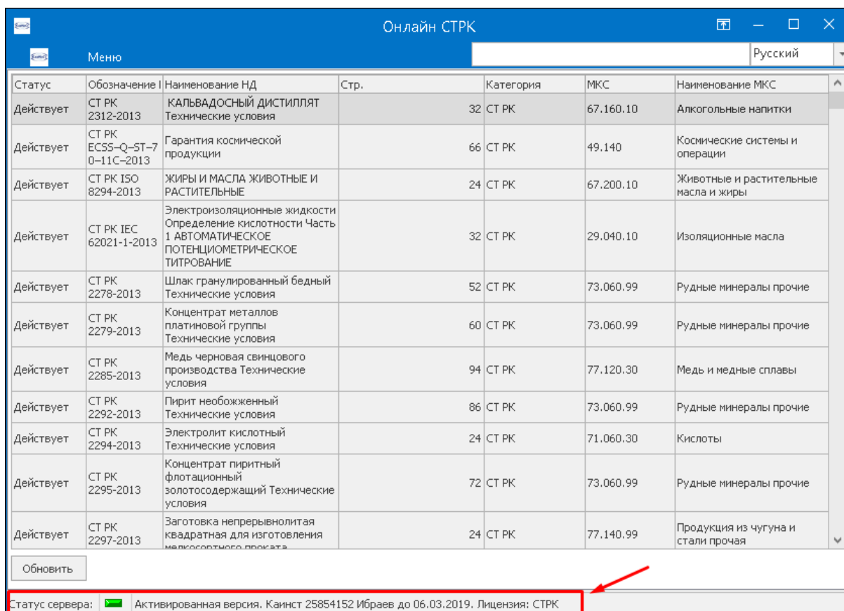
Рисунок 3 – активированная лицензия
